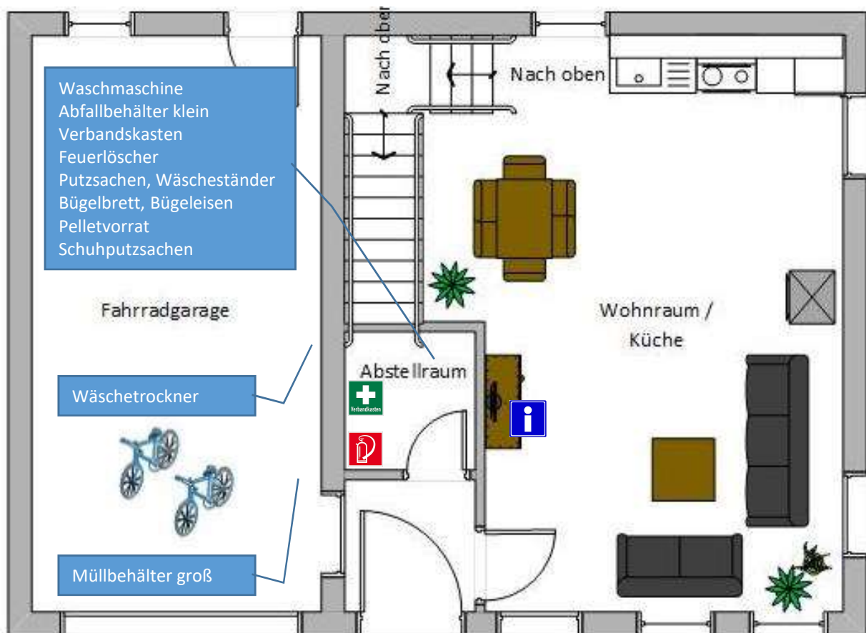
Grundriss Erdgeschoss
