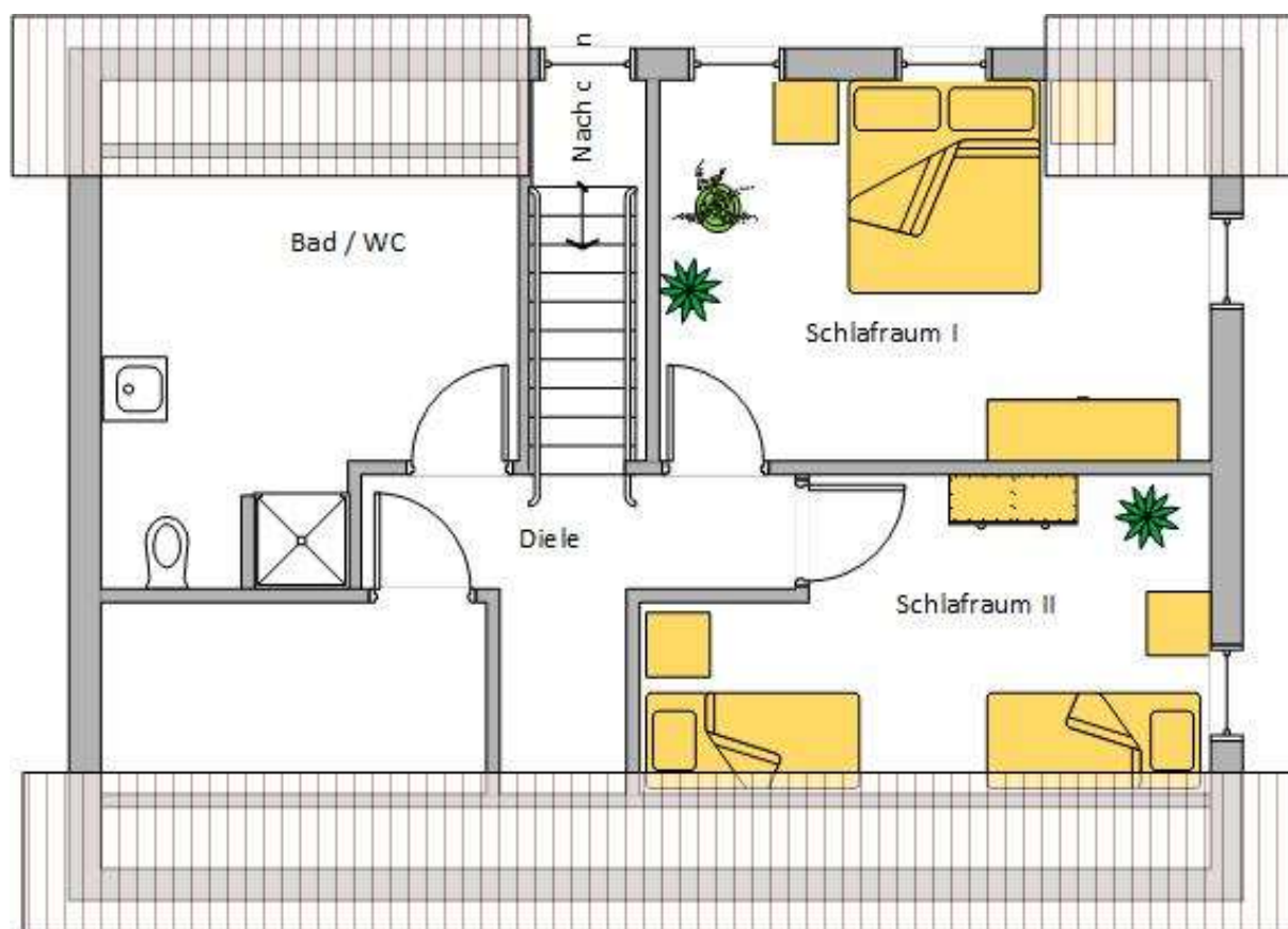
Grundriss Obergeschoss
